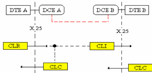
Fase di svincolo della chiamata (scambio di pacchetti Clear)
